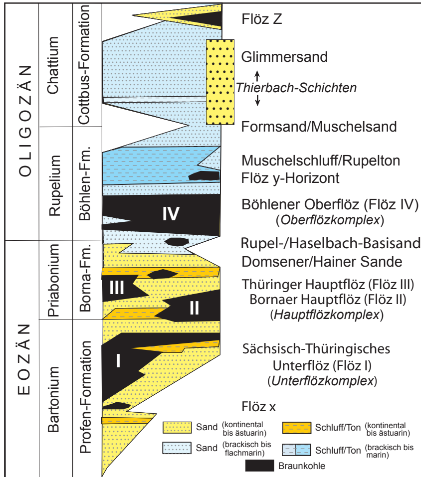
Abb. 23.10 Profilentwicklung im Bereich des Leipzig-Borna-Altener Tertiärgebietes ("Weißelster-Becken") (nach J. RASCHER et al. 2005; G. STANDKE 2008b; W. KRUTZSCH 2011)
