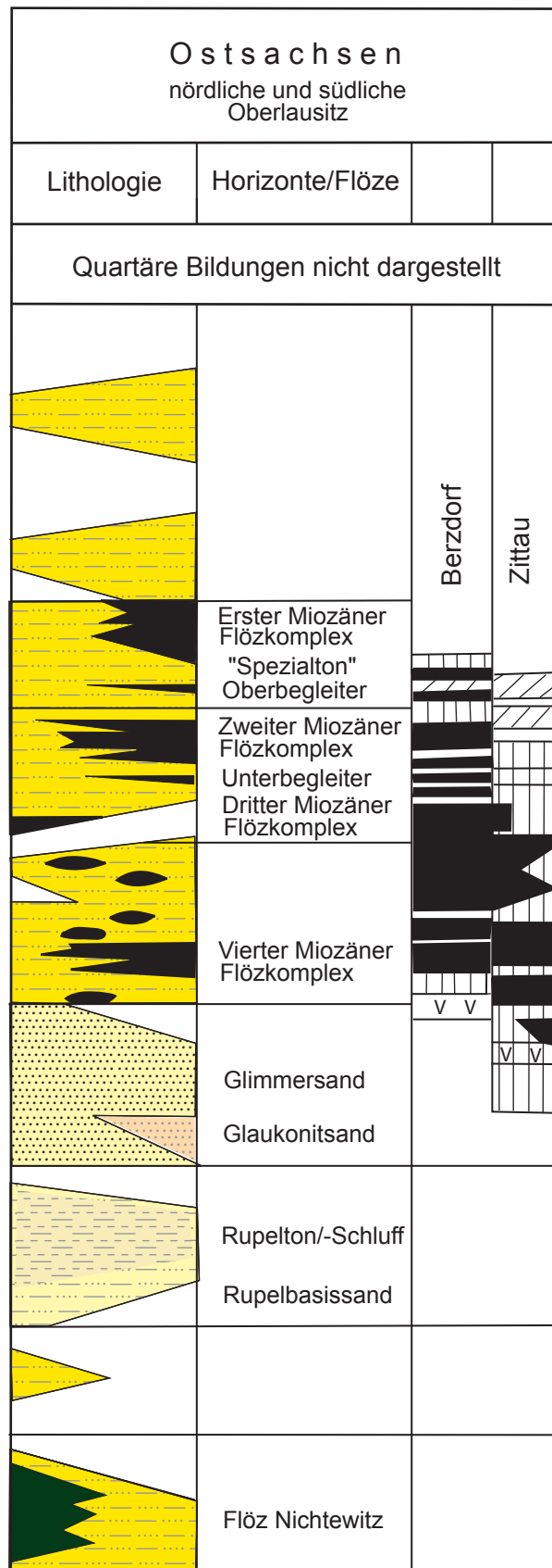
Abb. 23.12 Alter und Verbreitung der tertiären Braunkohlenflöze im Bereich Ostsachsens (nach J. RASCHER 2009)
