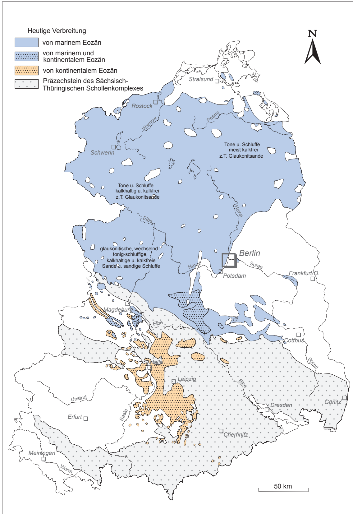
Abb. 23.2 Heutige Verbreitung von Ablagerungen des Eozän in Ostdeutschland (generalisierte Darstellung nach D. LOTSCH 1968; W. ALEXOWSKY 1994; J. HAUPT 1996; G. MARTIKLOS 2002a; D. LOTSCH 2002a; H. JORTZIG 2002a; W.v.BÜLOW & S. MÜLLER 2004; G. STANDKE 2008a, 2008b, 2015)
