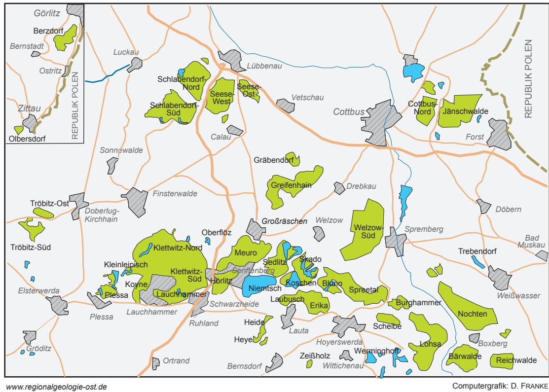
Abb. 23.6 Tagebaue (zumeist stillgelegt) des Lausitzer Braunkohlenreviers (im Wesentlichen nach W. NOWEL 1995)
