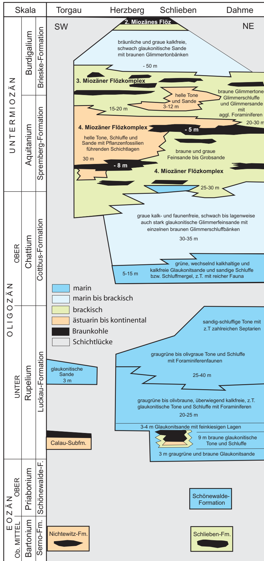
Abb. 23.8 Lithofazielle Profilentwicklung des Tertiär im Westabschnitt des Niederlausitzer Tertiärgebiets (schematische Darstellung nach D. LOTSCH et al. 1969; D. LOTSCH 1981, 2002b)
