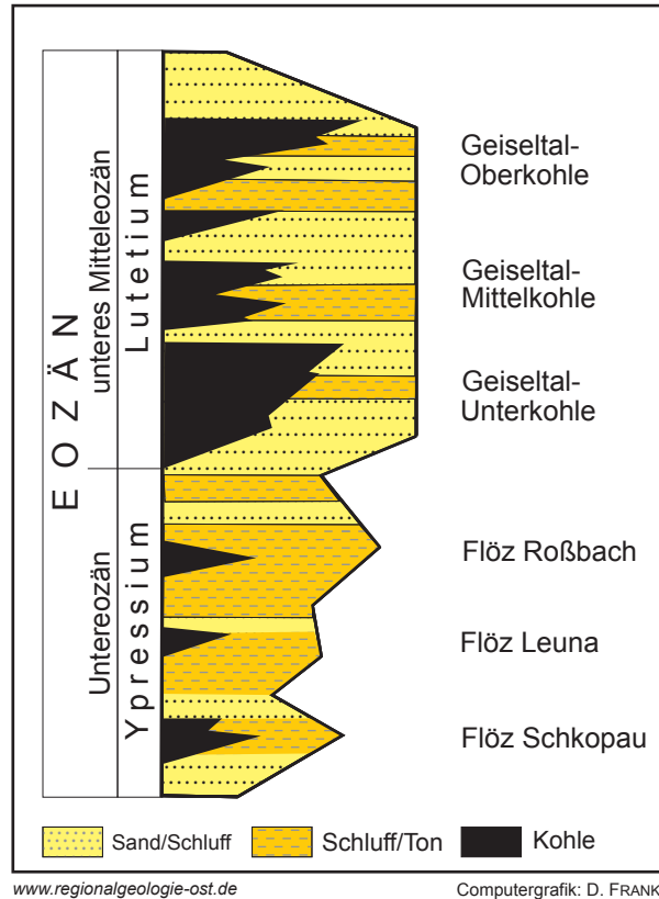
Abb. 23.9 Eozänprofil des Geiseltal-Beckens (nach J. RASCHER et al. (2005))
