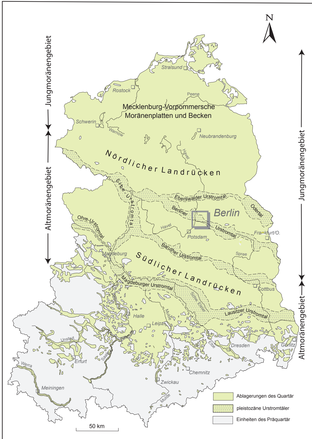
Abb. 24 Heutige Verbreitung von Ablagerungen des Quartär in Ostdeutschland (nach A.G. CEPEK 1976)
