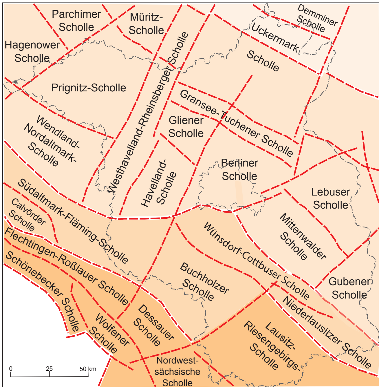
Abb. 25.12.1 Schollengliederung des Tafeldeckgebirges im Bereich des Landes Brandenburg (nach G. BEUTLER & W. STACKEBRANDT 2012)
