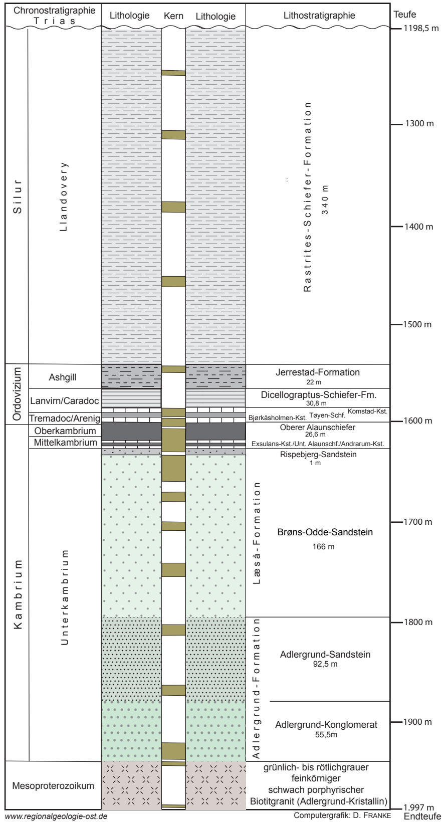
Abb. 25.15 Profil des Paläozoikum/Proterozoikum der Offshore-Bohrung G 14-1/86
