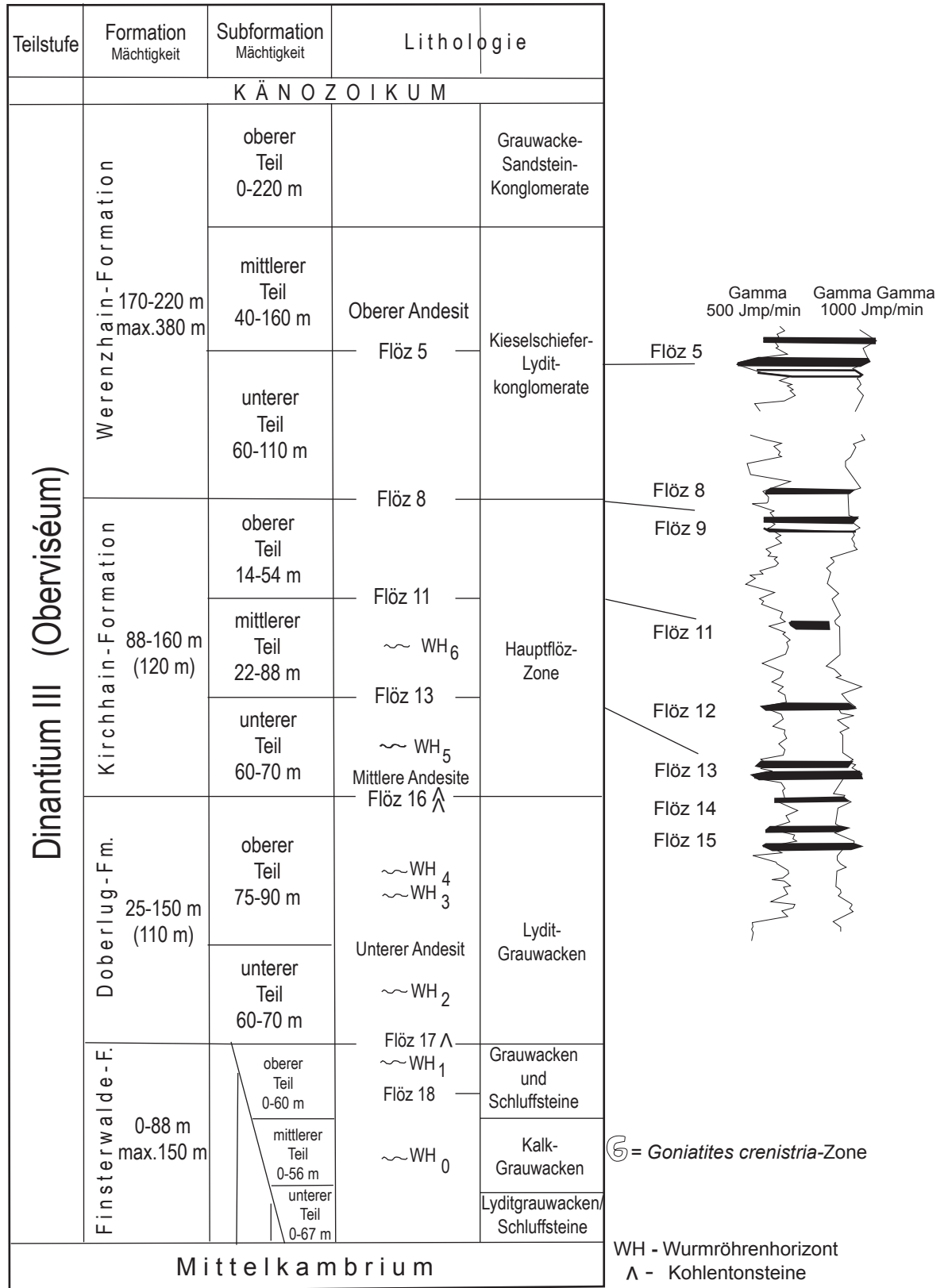
Abb. 25.19.1 Gliederung des Dinantium von Doberlug-Kirchhain (nach W. NÖLDEKE 1976, ergänzt von A. KAMPE 1998)
