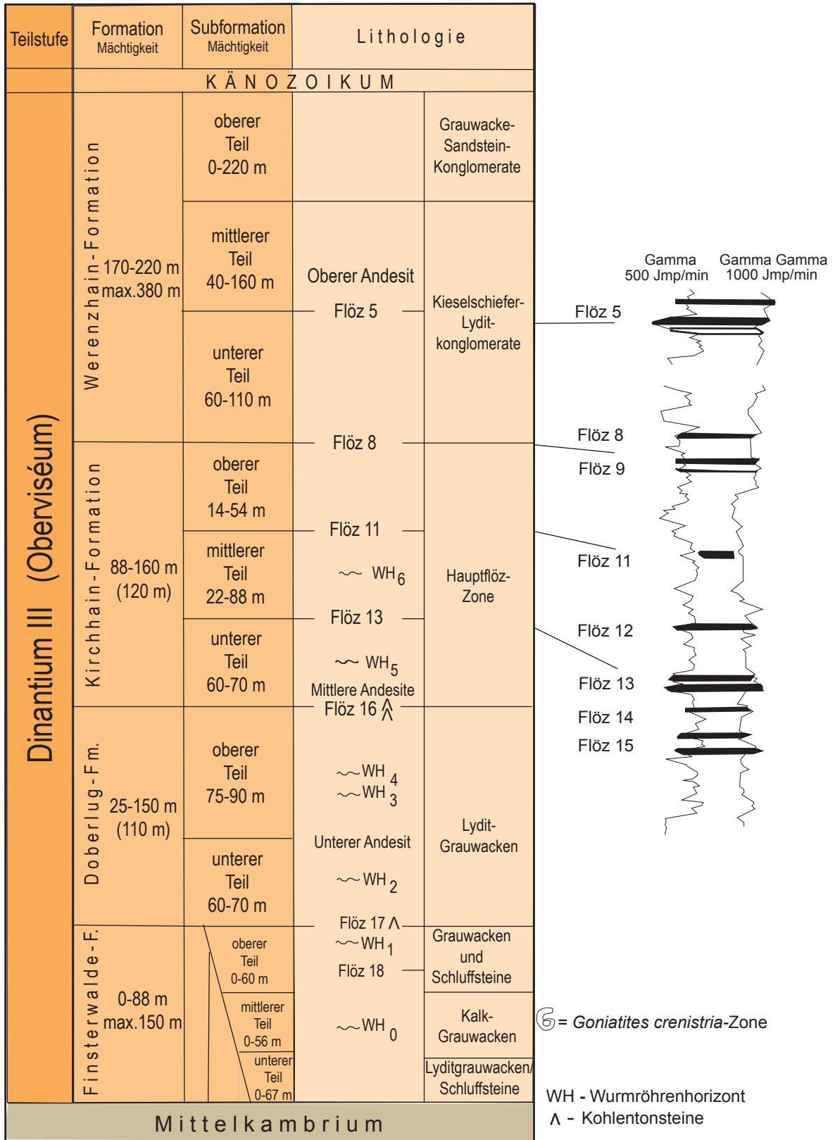
Abb. 25.19.1 Gliederung des Dinantium von Doberlug-Kirchhain (nach W. NÖLDEKE 1976, ergänzt von A. KAMPE 1988)
