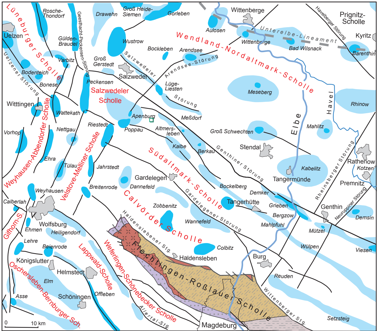
Abb. 25.20 Regionale Gliederung der Altmark-Fläming-Scholle und angrenzender Bereiche mit Darstellung der wichtigsten Salinarstrukturen (Salzstöcke dunkelblau, Salzklissen hellblau)
