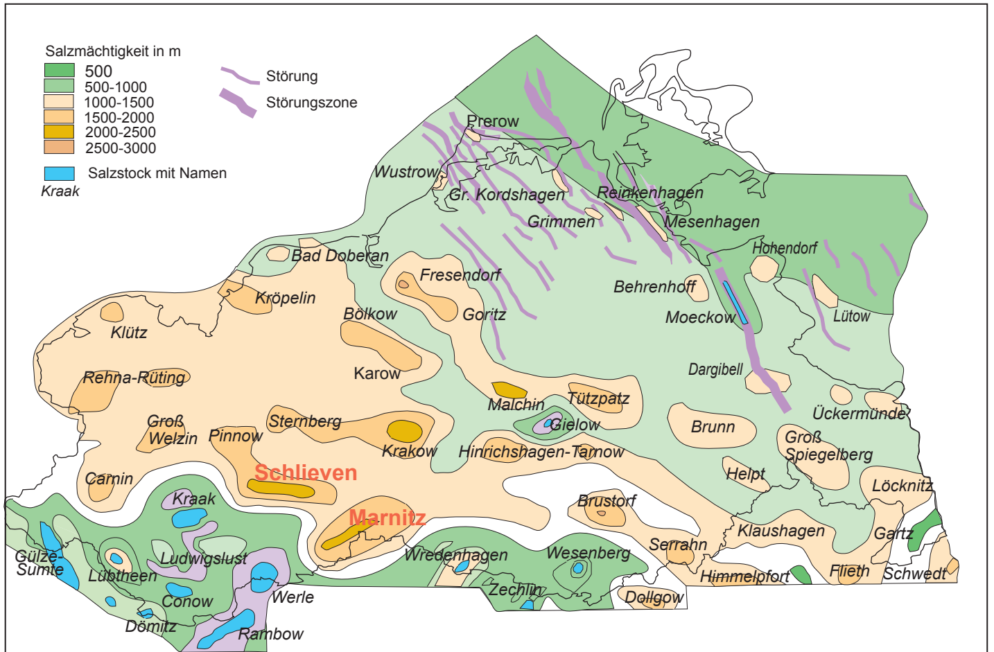
Abb. 25.21 Zechstein-Salzstrukturen in Mecklenburg-Vorpommern (nach N. RÜHBERG (1997); P. KRULL 2004a; U. MÜLLER & K. OBST 2008)
