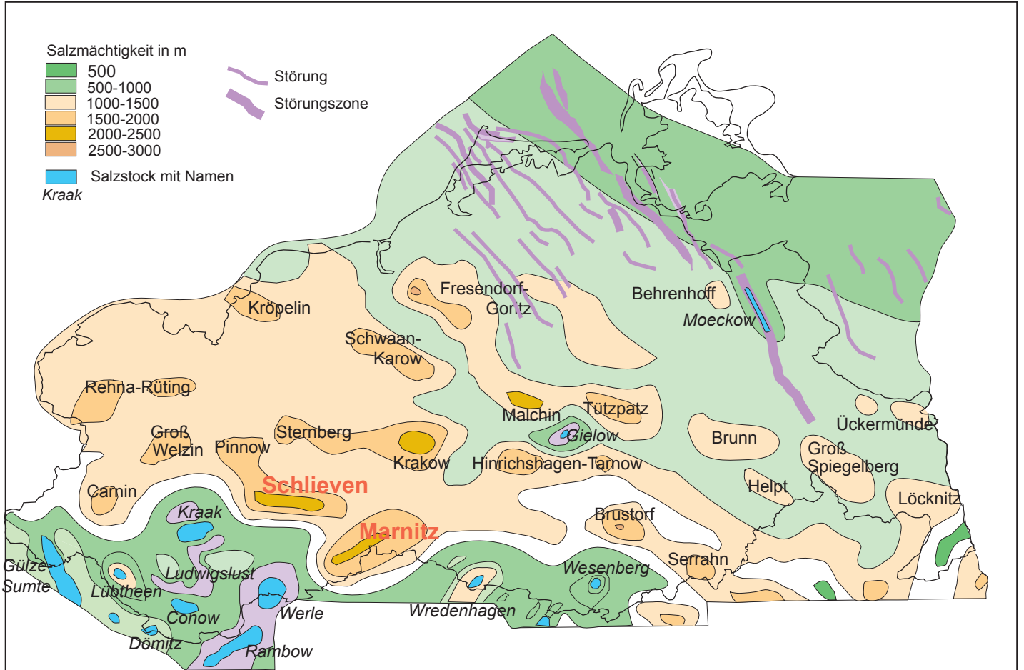
Abb. 25.21 Zechstein-Salzstrukturen in Mecklenburg-Vorpommern (nach U. MÜLLER & K. OBST 2008)
