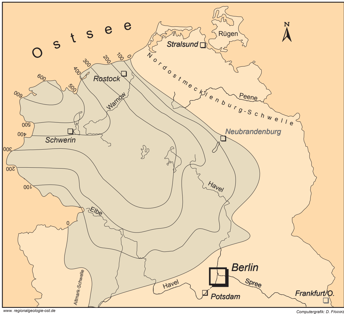
Abb. 25.25 Verbreitung und Mächtigkeit der Mirow-Formation des Rotliegenden im Bereich der Nordostdeutschen Senke
