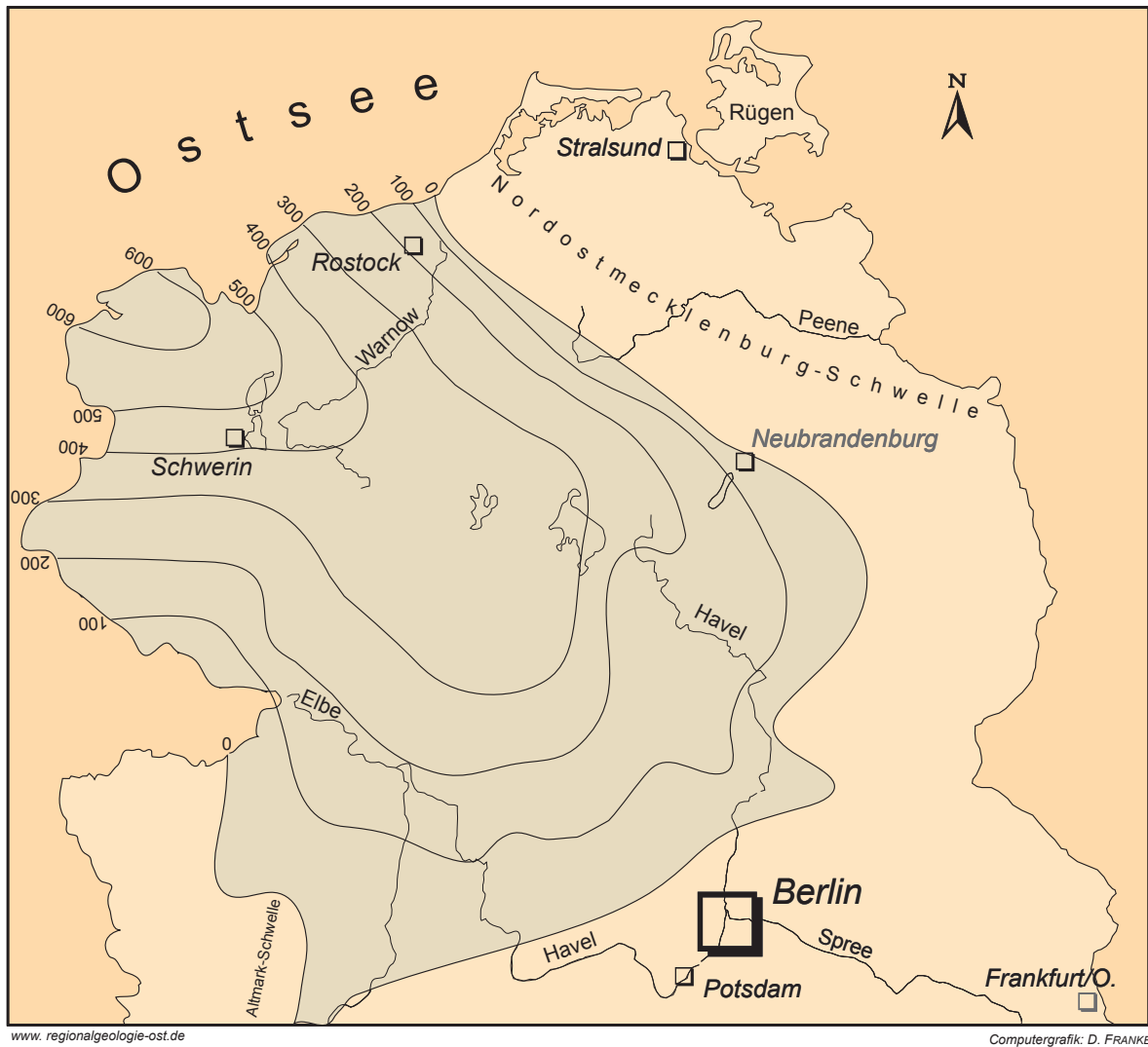
Abb. 25.25 Verbreitung und Mächtigkeit der Mirow-Formation des Rotliegend im Bereich der Nordostdeutschen Senke
