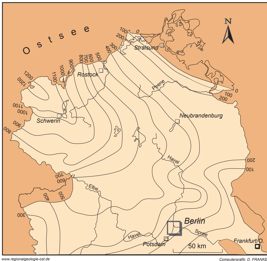
Abb. 25.26 Verbreitung und Mächtigkeit von Schichtenfolgen der Elbe-Subgruppe im Bereich der Nordostdeutschen Senke
