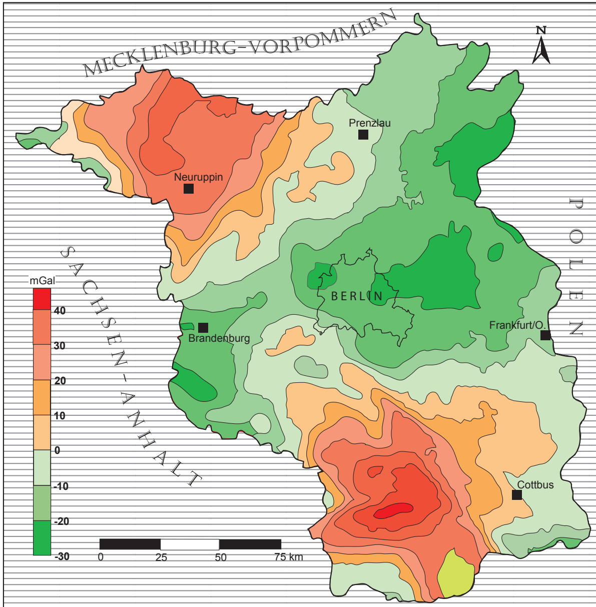
Abb. 25.33 Schwereanomalien (Bouguer-Anomalien) im Bereich des Landes Brandenburg (nach W. CONRAD 2010, R. GABRIEL et al. 2015)
