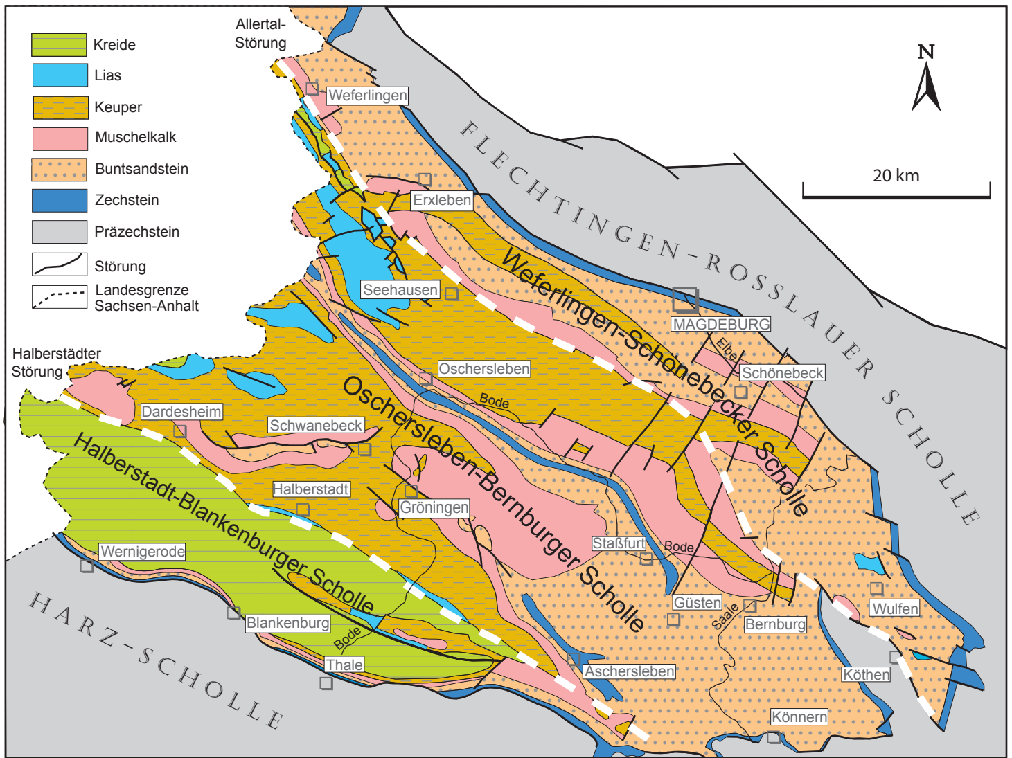
Abb. 28 Geologie der Subherzyna Senke Darstellung ohne känozoische Bildungen (nach G. MARTIKLOS et al. 2001)
