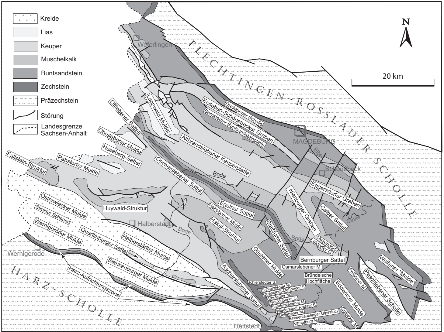
Abb. 28.1 Saxonischer Strukturbaue der Subhercynen Senke (nach I. KNAK & G. PRIMKE 1963; R. KUNERT & G. LENK 1964; TGL 34331/01 (1983); G. KATZUNG & G. EHMKE 1993; G. MARTIKLOS et al. 2001; G. BEUTLER 2001; G. PATZELT 2003; K.-H. RADZINSKI et al. 2008a) Zur Geologie der Subhercynen Senke vgl. Abb. 28, zum saxonischen Störungsmuster Abb. 28.2
