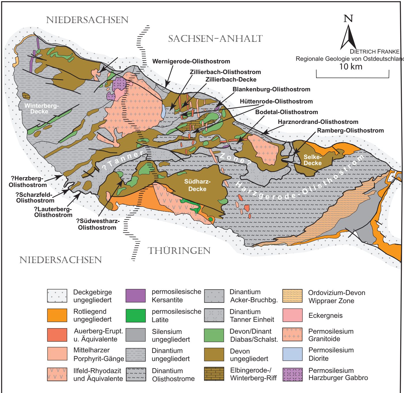
Abb. 29.2 Allochthone und olisthstromale Bildungen des Harzes (im Wörterbuch sind nur Begriffe des Osthazes enthalten) (nach H. LUTZENS & M. SCHWAB 1972; C. HINZE et al. 1998; G. MARTIKLOS et al. 2001; M. SCHWAB 2008a)
