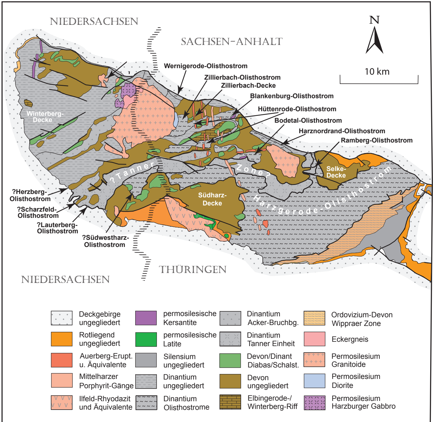
Abb. 29.2 Allochthone und olistostromale Bildungen des Harzes (im Wörterbuch sind nur Begriffe des Ostharzes enthalten) (nach H. LUTZENS & M. SCHWAB 1972; C. HINZE et al. 1998; G. MARTIKLOS et al. 2001; M. SCHWAB 2008a)
