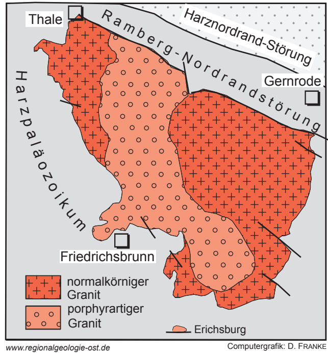
Abb. 29.6 Geologie des Ramberg-Plutons (nach R. BENEK 1967, C. HINZE et al. 1998)
