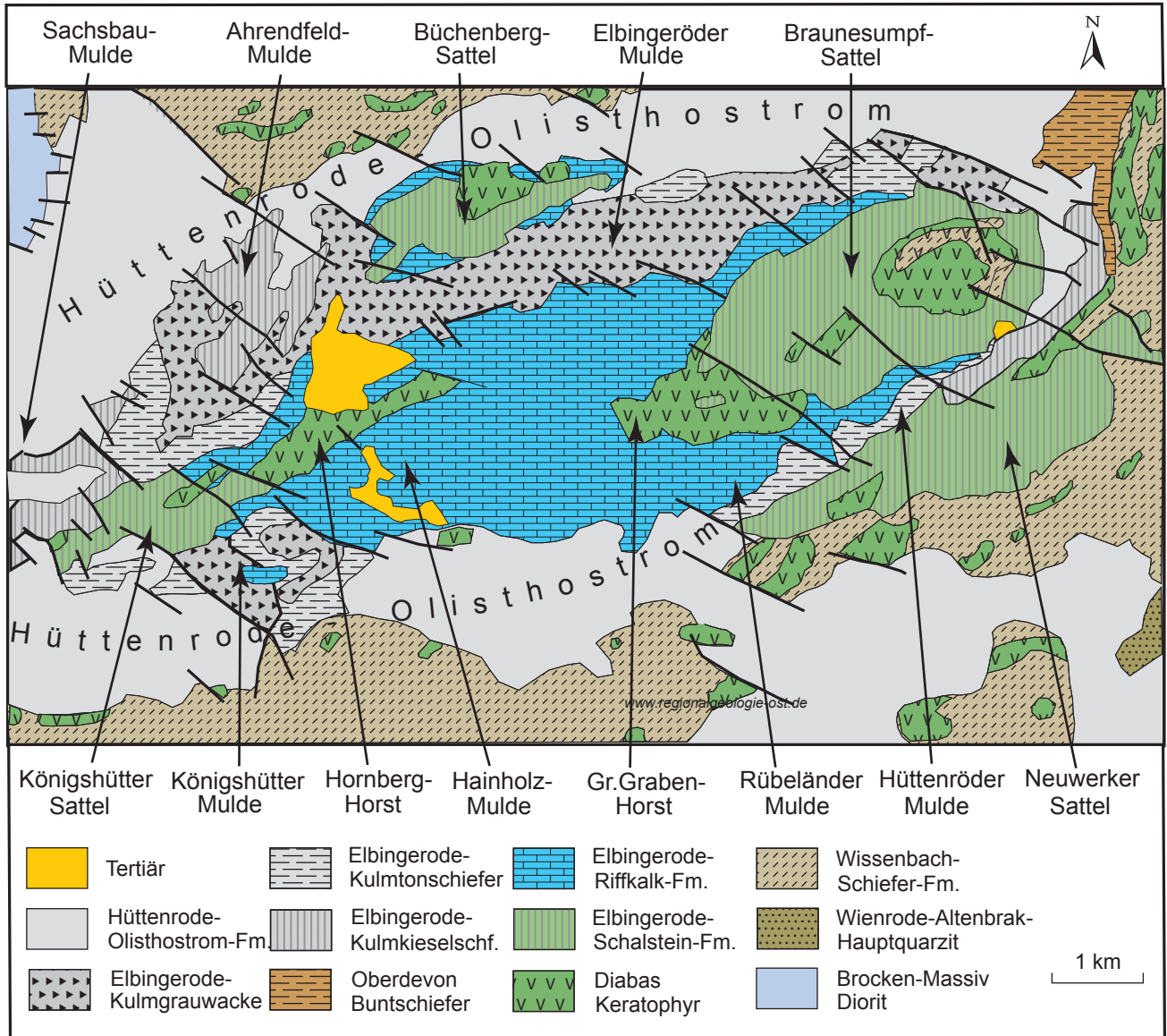
Abb. 29.7 Geologie des Elbingeröder Komplexes Darstellung ohne Mittelharzer Eruptivgesteinsgänge (nach H. LUTZENS 1979; K. RUCHHOLZ & H. WELLER 1988, 1991a; C. HINZE et al. 1998; G. MEYENBURG 2017)
