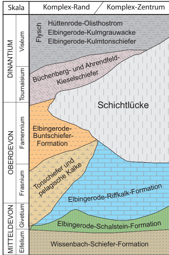
Abb. 29.8 Profilentwicklung im Bereich des Elbingeröder Komplexes (nach K.-H. BORSDORF et al. 1973; H. WELLER 1991b; C.-H. FRIEDEL 1995)
