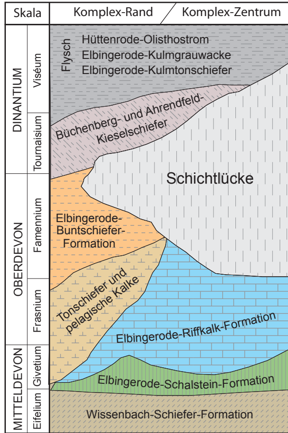
Abb. 29.8 Profilentwicklung im Bereich des Elbingeröder Komplexes (nach K.-H. BORSCHORF et al. 1973; H. WELLER 1991b; C.-H. FRIEDEL 1995)
