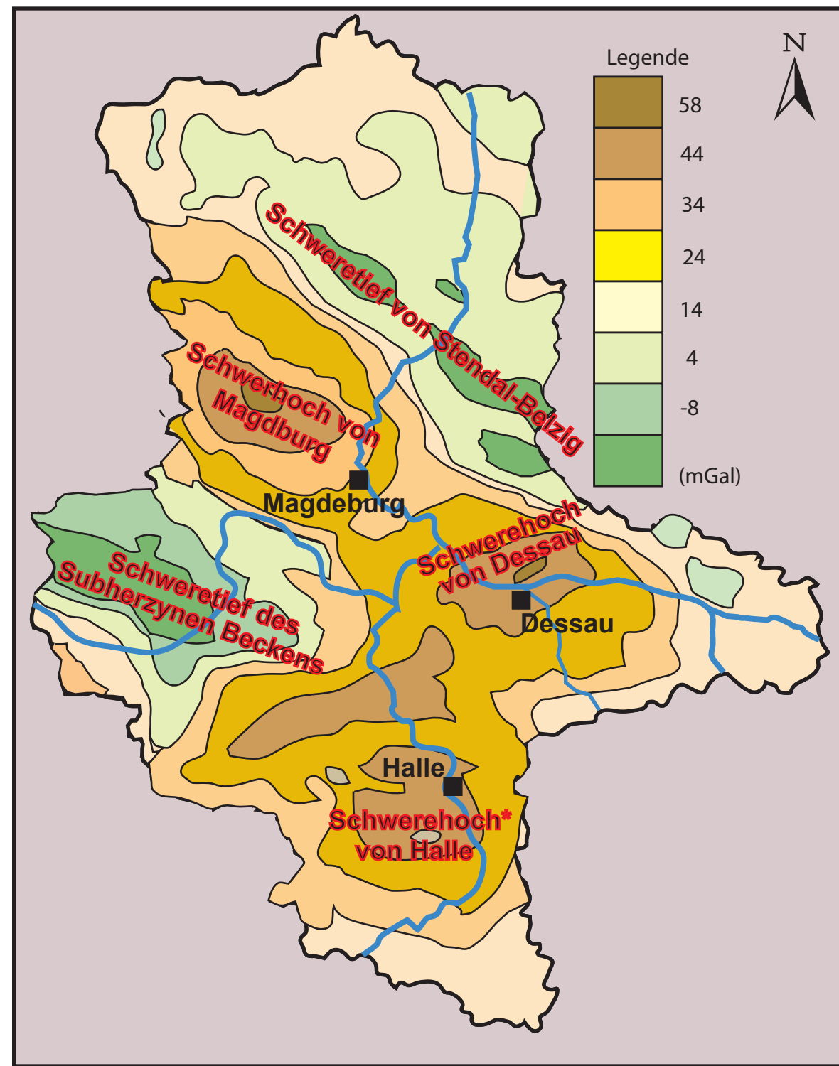
Abb. 30.13.3 Gravimetrische Übersichtskarte von Sachsen-Anhalt nach W. KNOTH, U. KRIEBEL & W. LANGE (1996); W. LANGE & I. RAPPILBER (2008)
