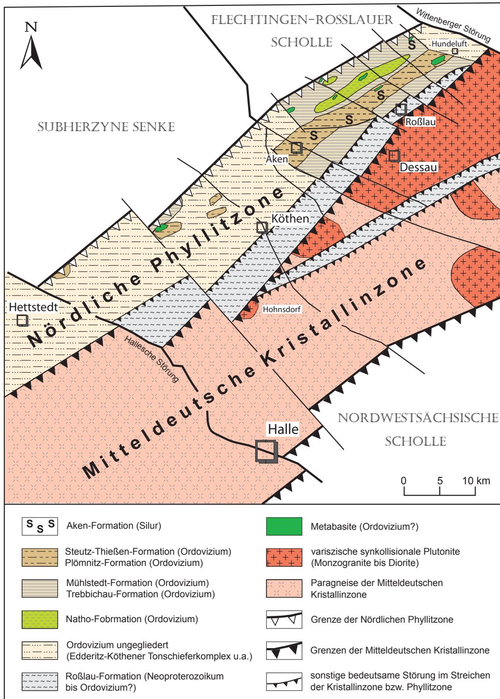
Abb. 30.3 Verbreitung und Ausbildung des Vor- und Altpaläozoikum unter permokarbonischer und jüngerer Bedeckung im Bereich zwischen Subherzyner Senke/Flechtingen-Roßlauer Scholle und Nordwestsächsischer Scholle
