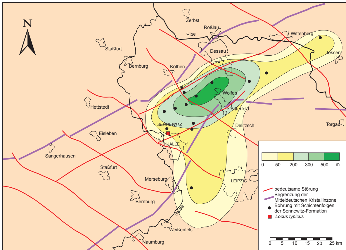
Abb. 30.8 Potentielle Verbreitung und Mächtigkeit von Schichtenfolgen der Sennewitz-Formation im Bereich der nordöstlichen Saale-Senke (nach I. RAPPILBER 2003)
