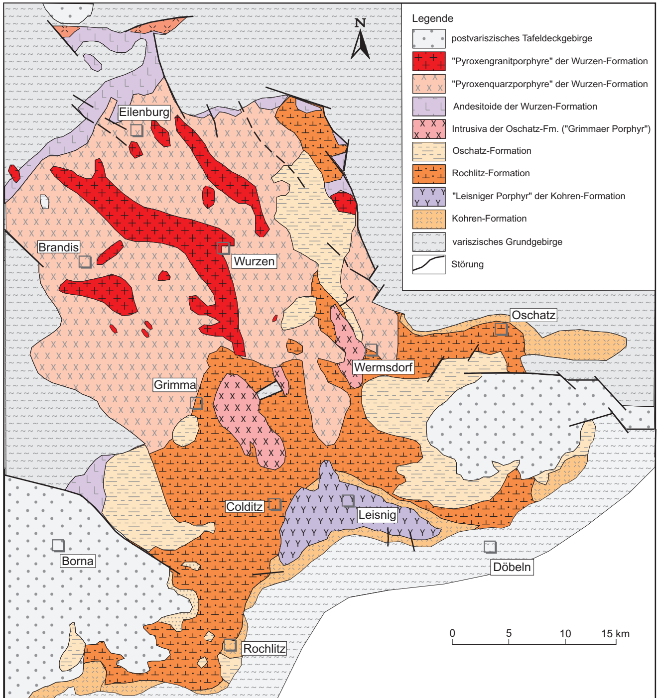
Abb. 31 Geologie des Nordwestsächsischen Eruptivkomplexes Darstellung ohne kanozoische Bildungen
