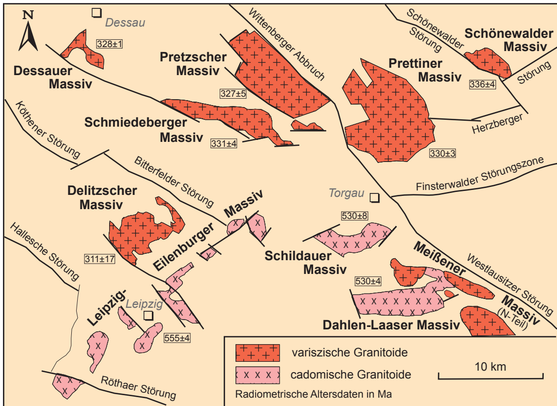
Abb. 31.1 Granitoid-Vorkommen in NW-Sachsen und im südöstlichen Sachsen-Anhalt (aus B. RÖBER et al. 1998)
