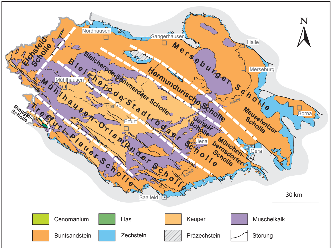
Abb. 32.1 Schollengliederung des Thüringer Beckens sensu lato Darstellung ohne känozoische Bildungen
