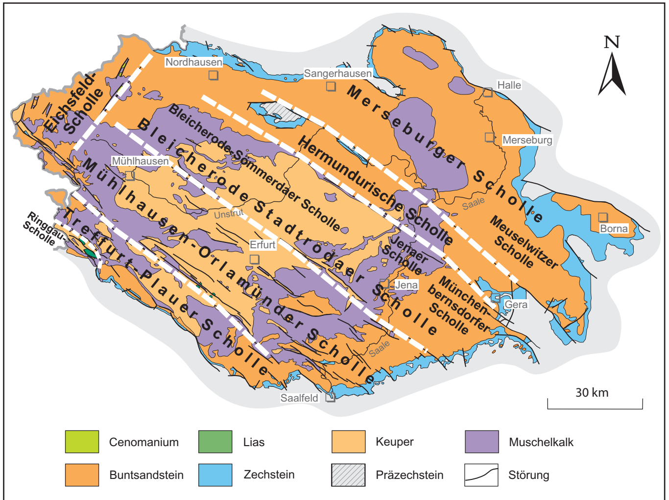
Abb. 32.1 Schollengliederung des Thüringer Beckens sensu lato Darstellung ohne känozoische Bildungen (nach Geologie-Standard TGL 34331/01 1983; G. KATZUNG & G. EHMKE/Hrsg. 1993; G. SEIDEL 2003, 2004)
