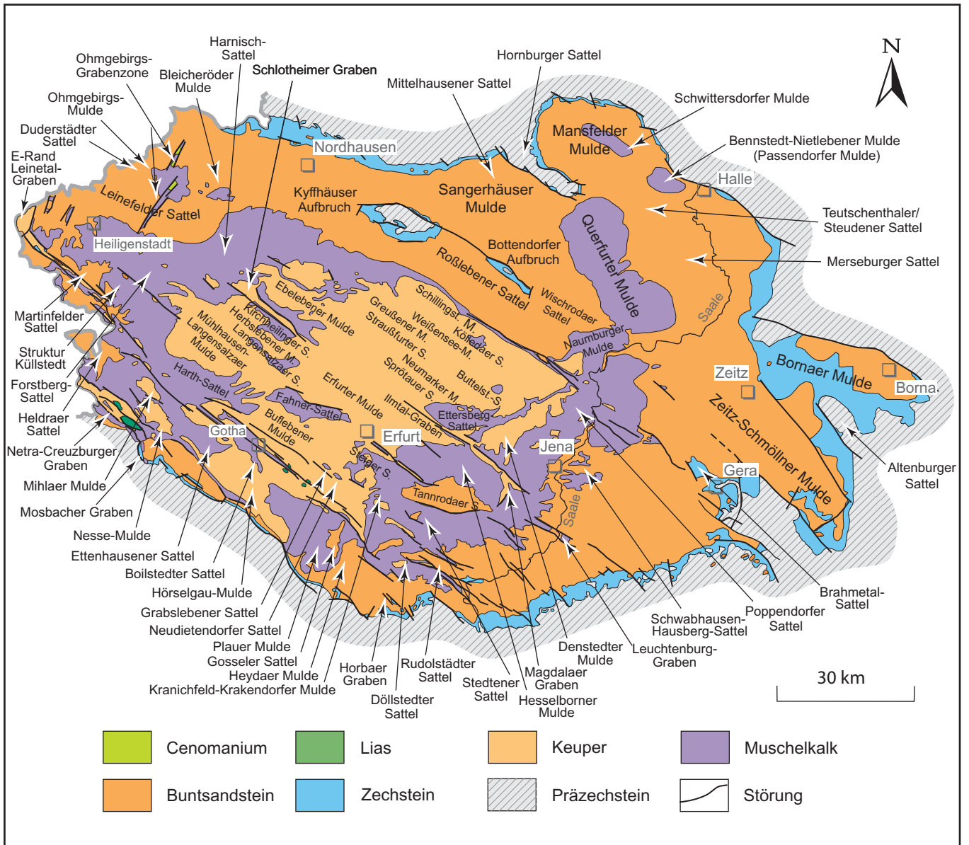
Abb. 32.2 Saxonische Strukturen im Bereich des Thüringer Beckens sensu lato (Auswahl) Darstellung ohne känozoische Bildungen (nach G. SEIDEL et al. 2002; I. RAPPILBER 2003; G. SEIDEL 2003, 2004)
