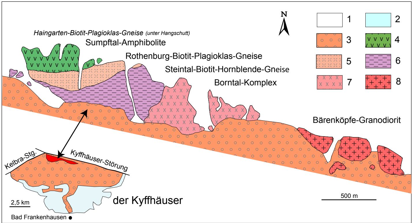
Abb. 32.5 Geologie des Kyffhäuser-Kristallins (nach A. ZEH & J. WUNDERLICH 2003; A. ZEH 2003; H.J. FRANZKE et al. 2007)
