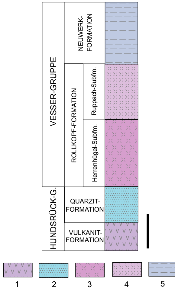
Abb. 33.3 Stratigraphie des Kambrium im Bereich der Schiefergebirgsinsel von Schmiedefeld-Vesser
