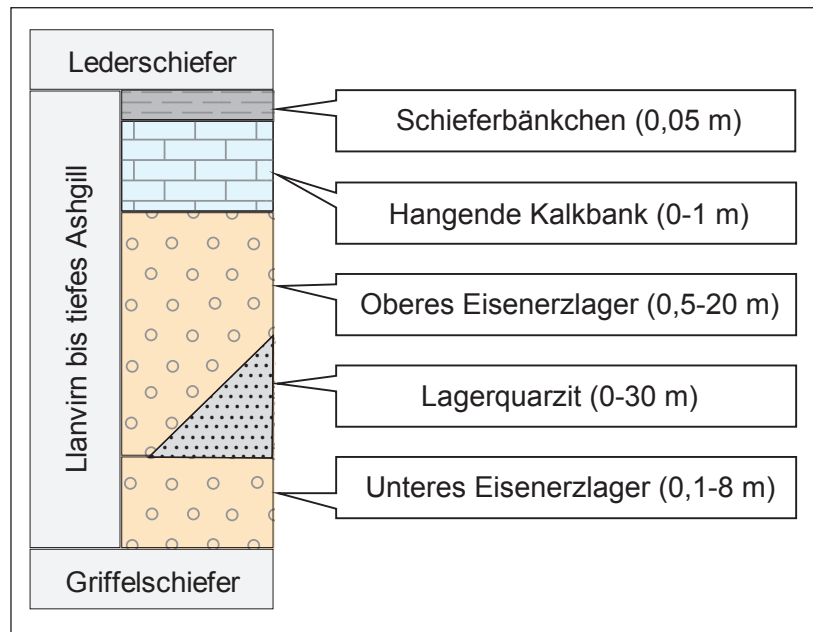
Abb. 34.4 Kondensiertes Profil des Llanvirn bis tiefen Ashgill (Schmiedefeld-Formation) an der SE-Flanke des Schwarzbürger Antiklinoriums
