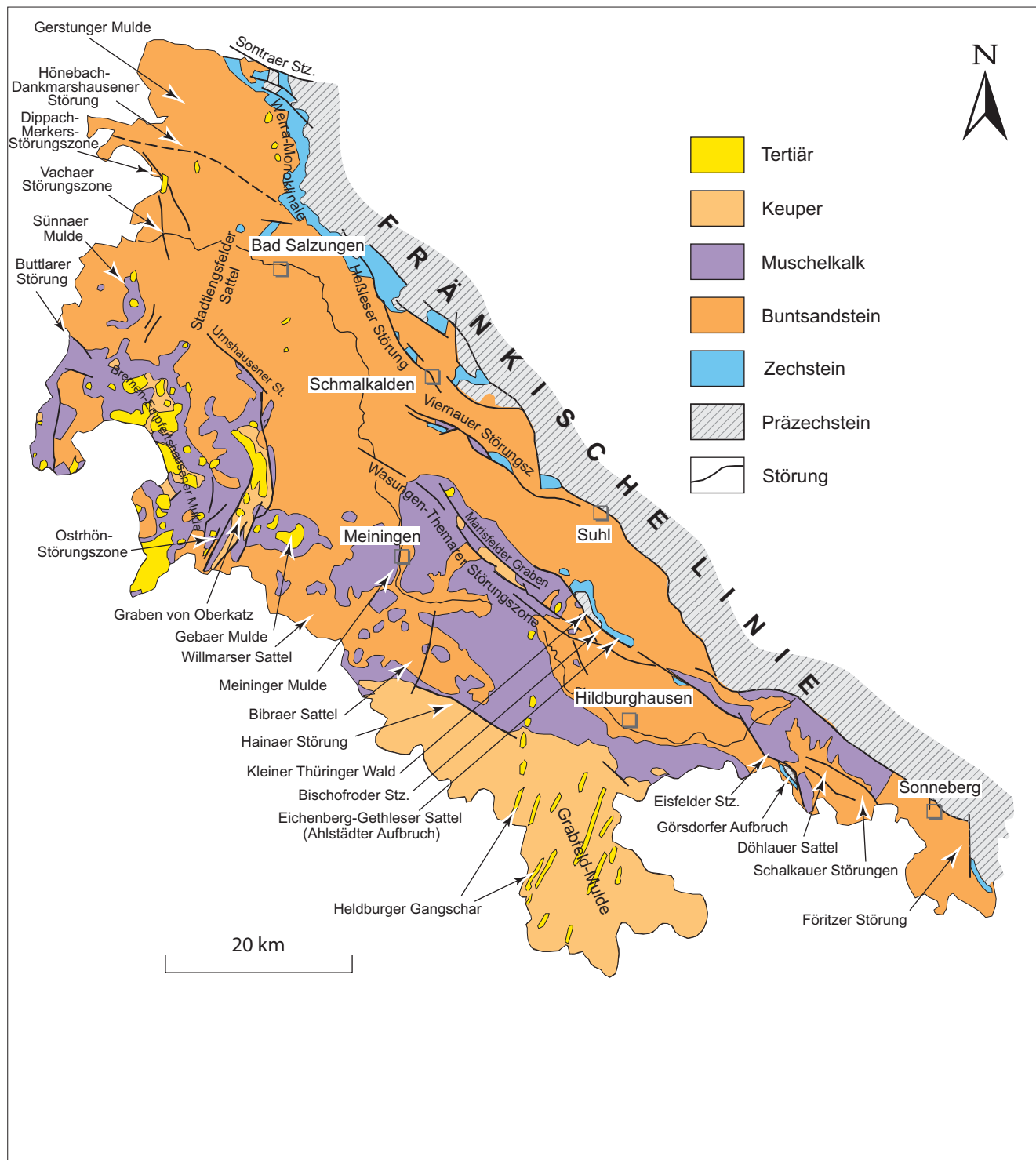
Abb. 35.2 Saxonische Strukturelemente im Bereich der Thüringisch-Fränkischen Scholle (Auswahl) Darstellung ohne Sedimente des Känozoikum
