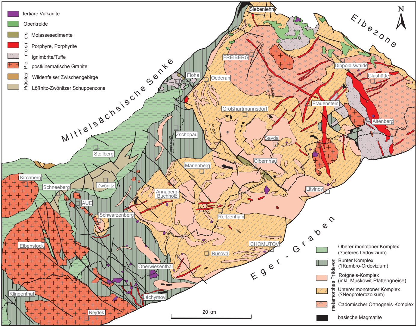
Abb. 36 Geologie des Erzgebirgs-Antiklinoriums
