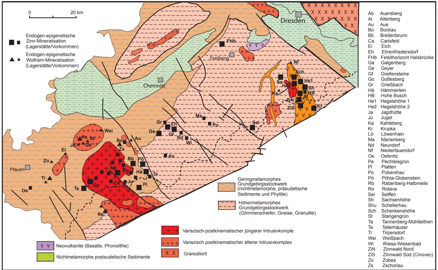
Abb. 36.11 Zinn- und Wolfram-Mineralisationen im Bereich von Sachsen (nach G. HÖSEL et al. 2009)
