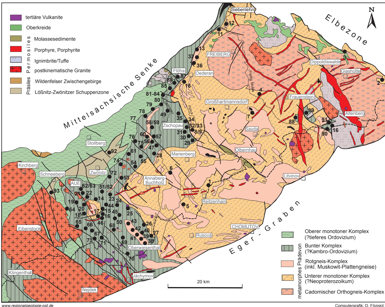
Abb. 36.14.1 Marmor-Vorkommen im Bereich des Erzgebirgs-Antiklinoriums (deutscher Anteil)
