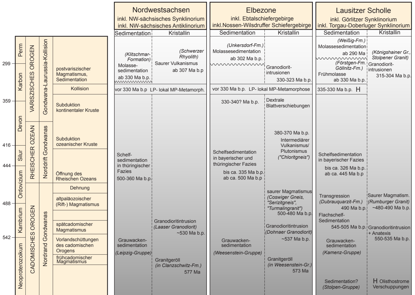
Abb. 36.16 Cadomisch-variszische Entwicklung im Nordost-Abschnitt der Saxothuringischen Zone
