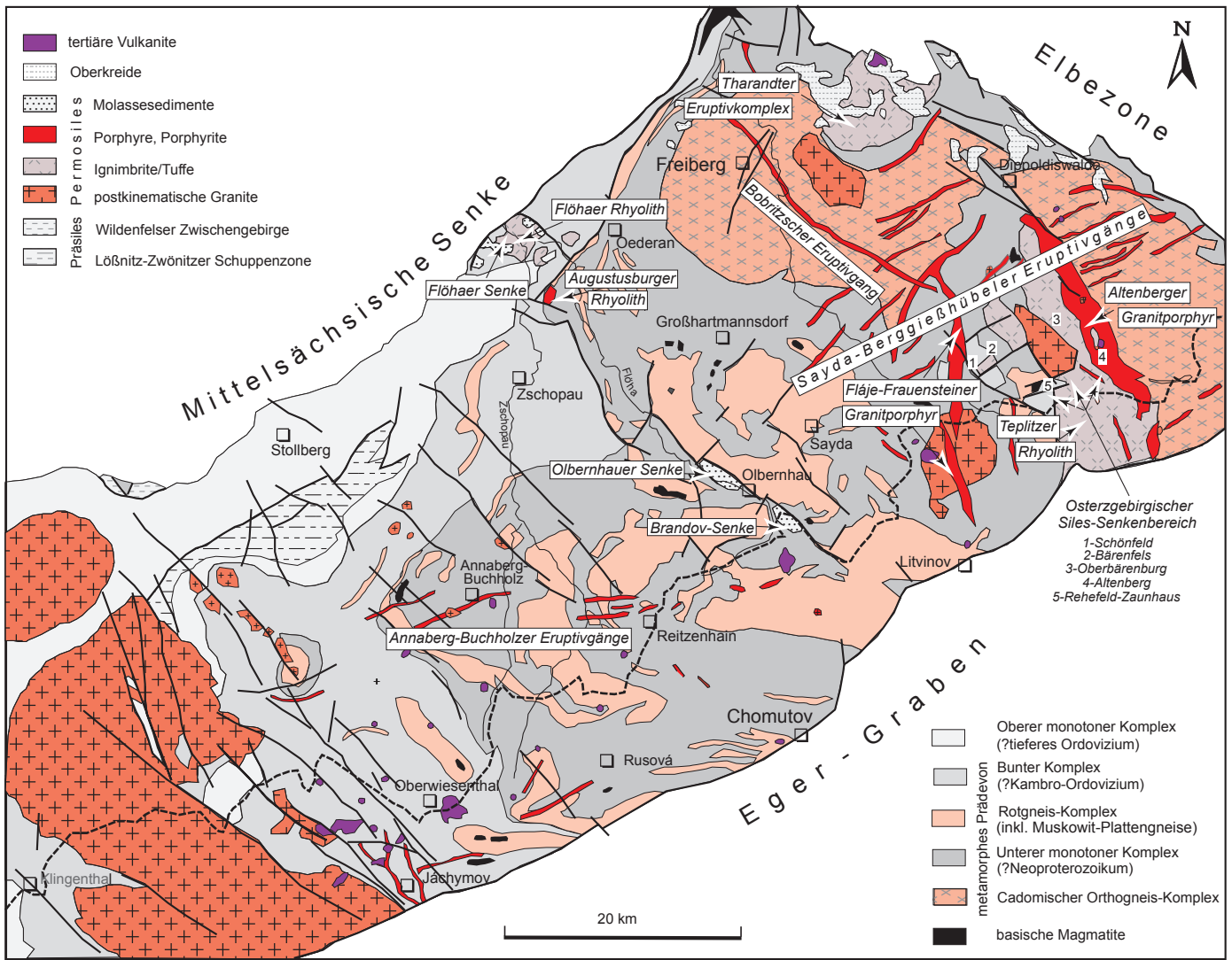
Abb. 36.3 Permosilesische Eruptiva und Molassevorkommen im Bereich des Erzgebirgs-Antiklinoriums
