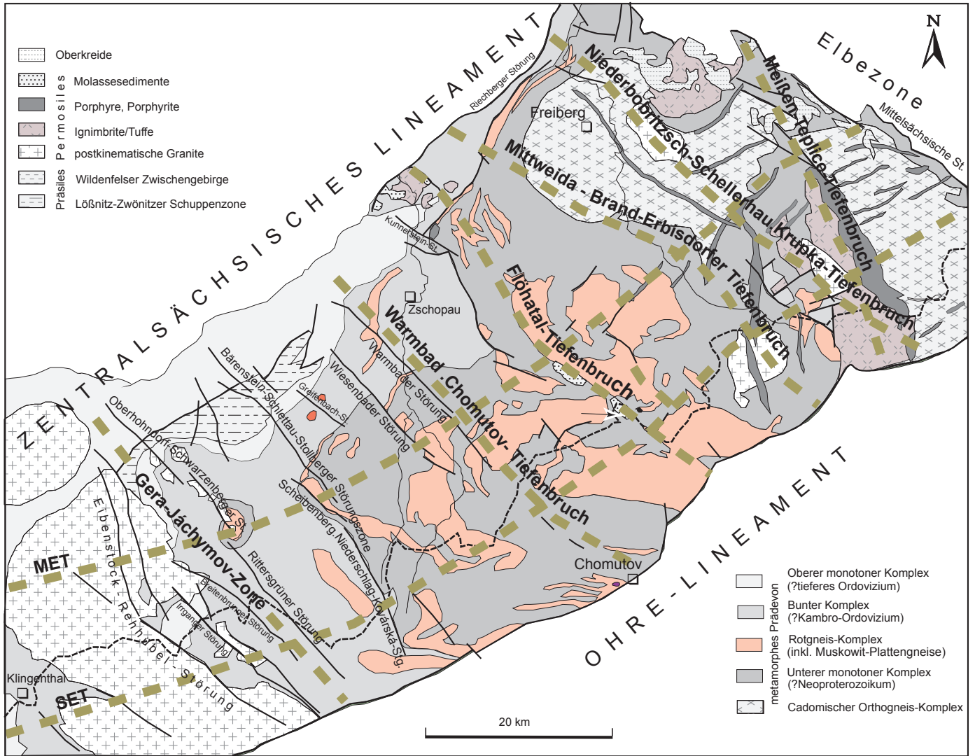
Abb. 36.4 Bedeutsame Störungen im Bereich des Erzgebirgs-Antiklinoriums
