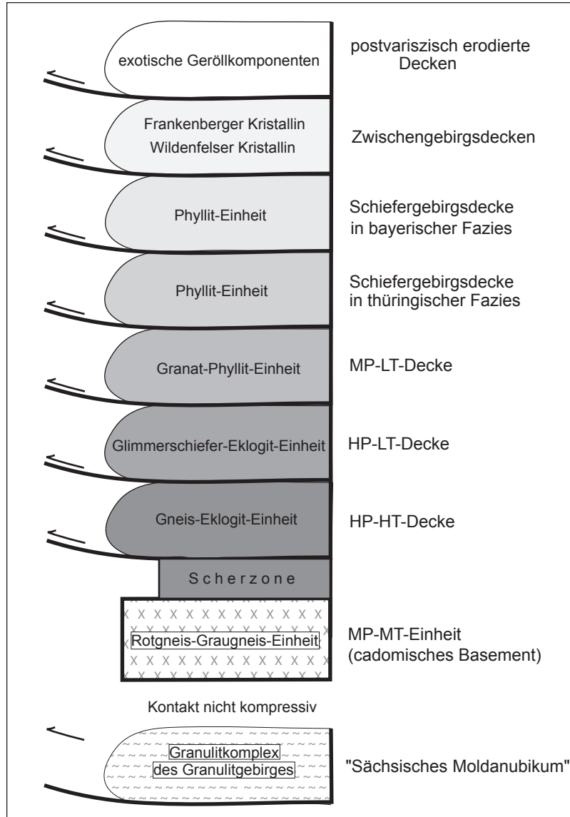
Abb. 36.5 Modell der Deckenstapelung im östlichen Saxothuringikum (nach K. RÖTZLER 1995; U. KRONER & U. SEBASTIAN 1997; B. MINGRAM & K. RÖTZLER 1999; K. RÖTZLER & B. PLESSEN 2010)
