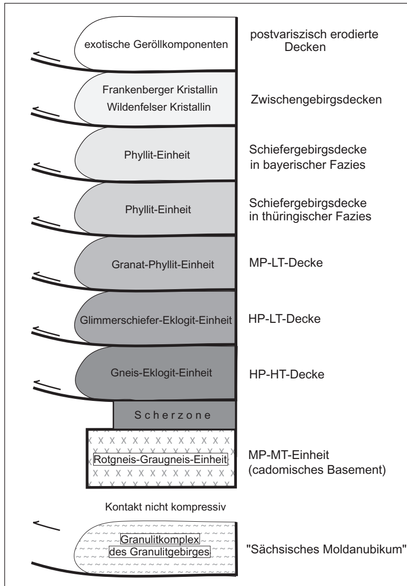
Abb. 36.5 Modell der Deckenstapelung im östlichen Saxothuringikum (nach K. RÖTZLER 1995; U. KRONER & U. SEBASTIAN 1997; B. MINGRAM & K. RÖTZLER 1999)
