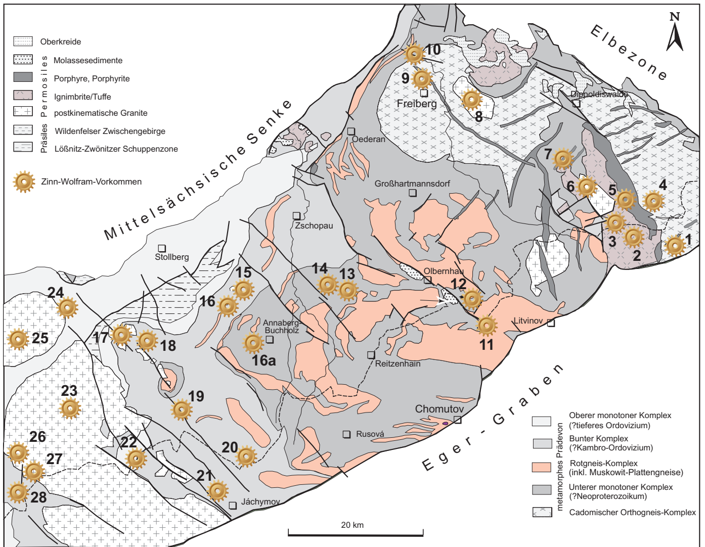
Abb. 36.6 Regionale Verbreitung variszischer Zinn-Wolfram-Vorkommen im Erzgebirge (Auswahl)
