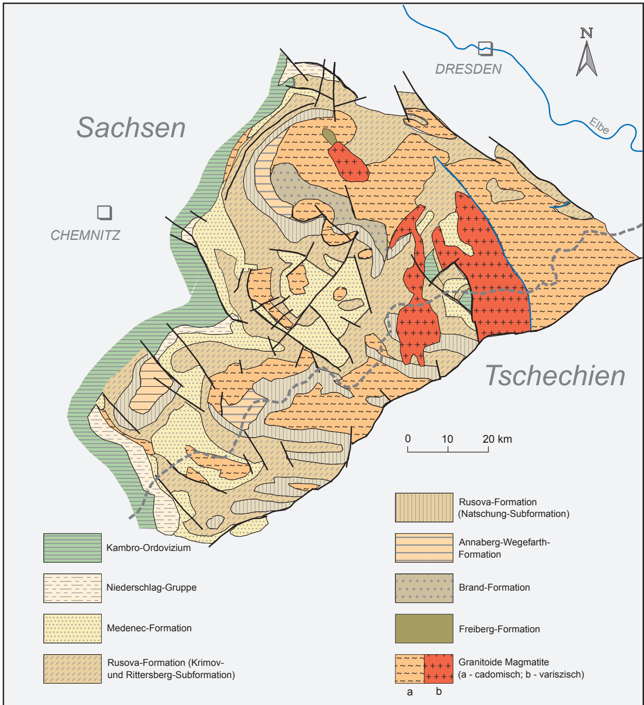
Abb.. 36.9 Regionale Verbreitung lithologischer Kartierungseinheiten des Proterozoikum im Bereich des Erzgebirgs-Antiklinoriums Darstellung ohne postkarbonische Bildungen
