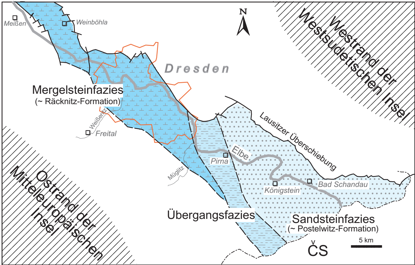
Abb. 39.3 Paläogeographie des Turonium/Coniacium der Elbtalkreide (hier: Räcknitz-Formation, mittelturone Übergangsfazies, Postelwitz-Formation) mit annähernd homogener Beckenkonfiguration bei regional differenzierter Lithofaziesentwicklung
