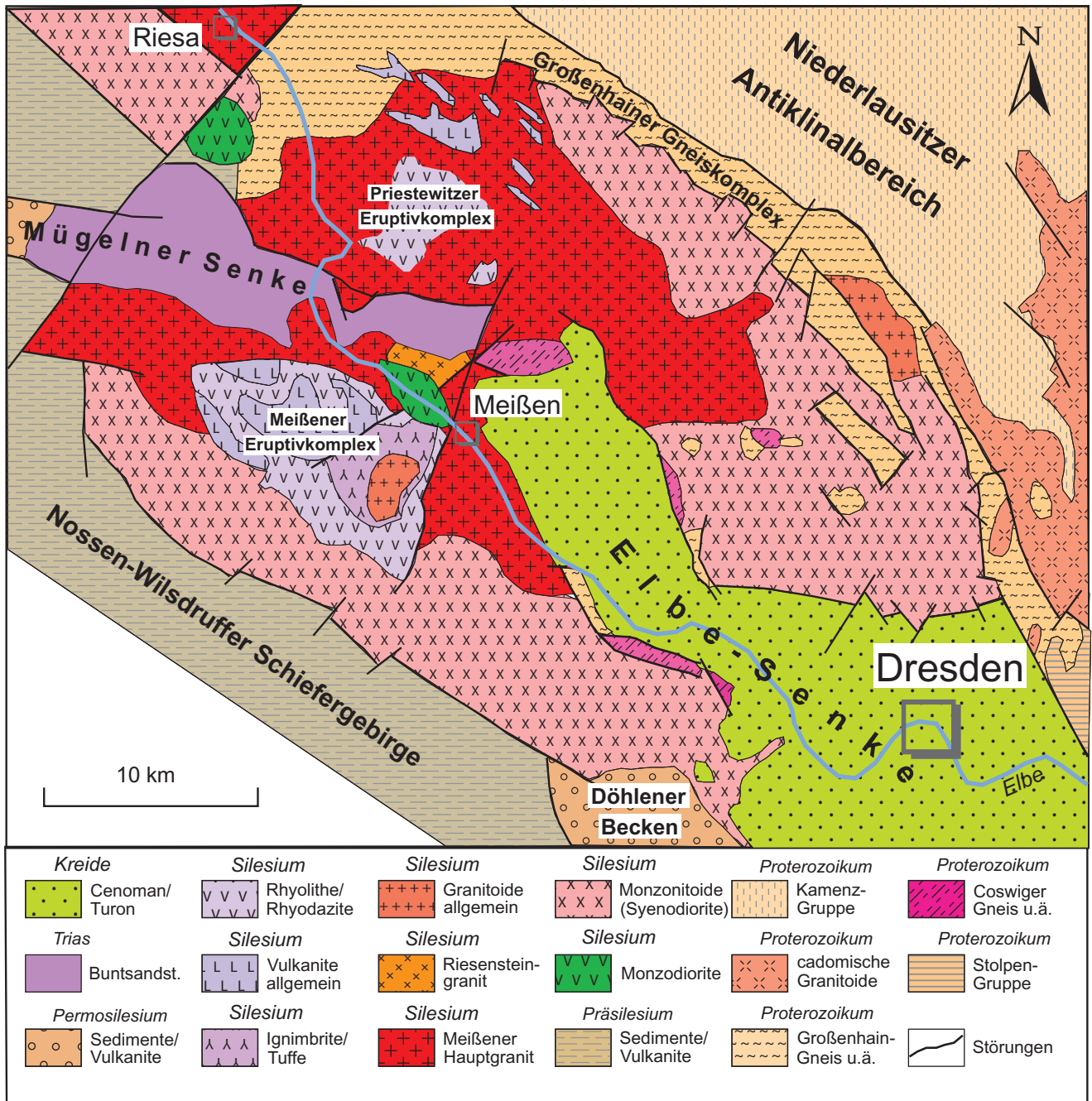
Abb. 39.4 Geologie des Meißener Massivs Darstellung ohne känozoische Bildungen
