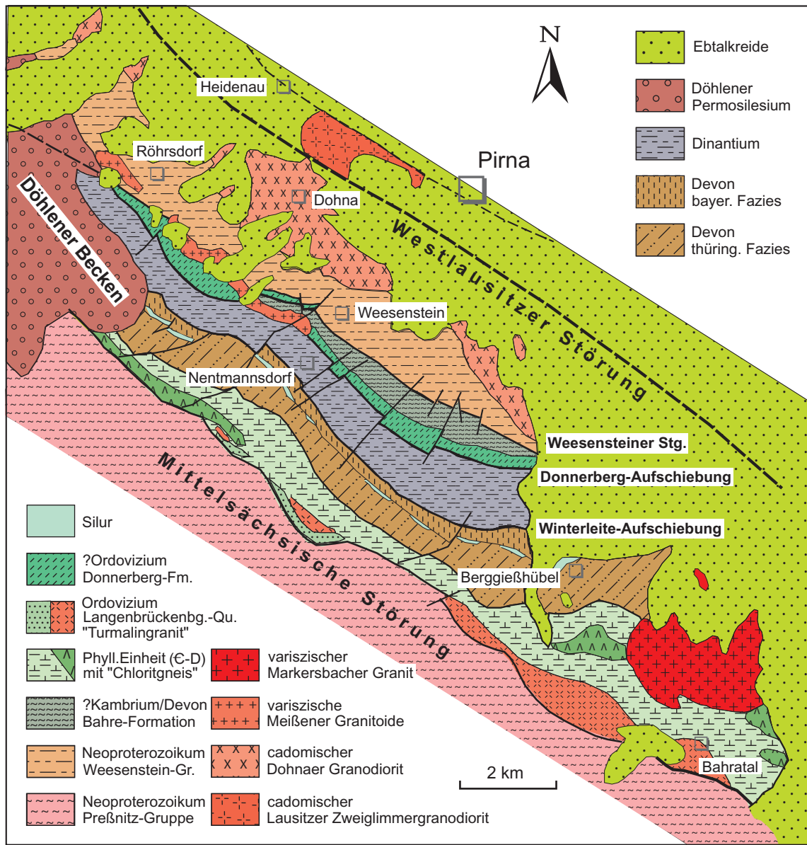
Abb. 39.7 Geologie des Elbtalschiefergebirges Darstellung ohne känozoische Bildungen
