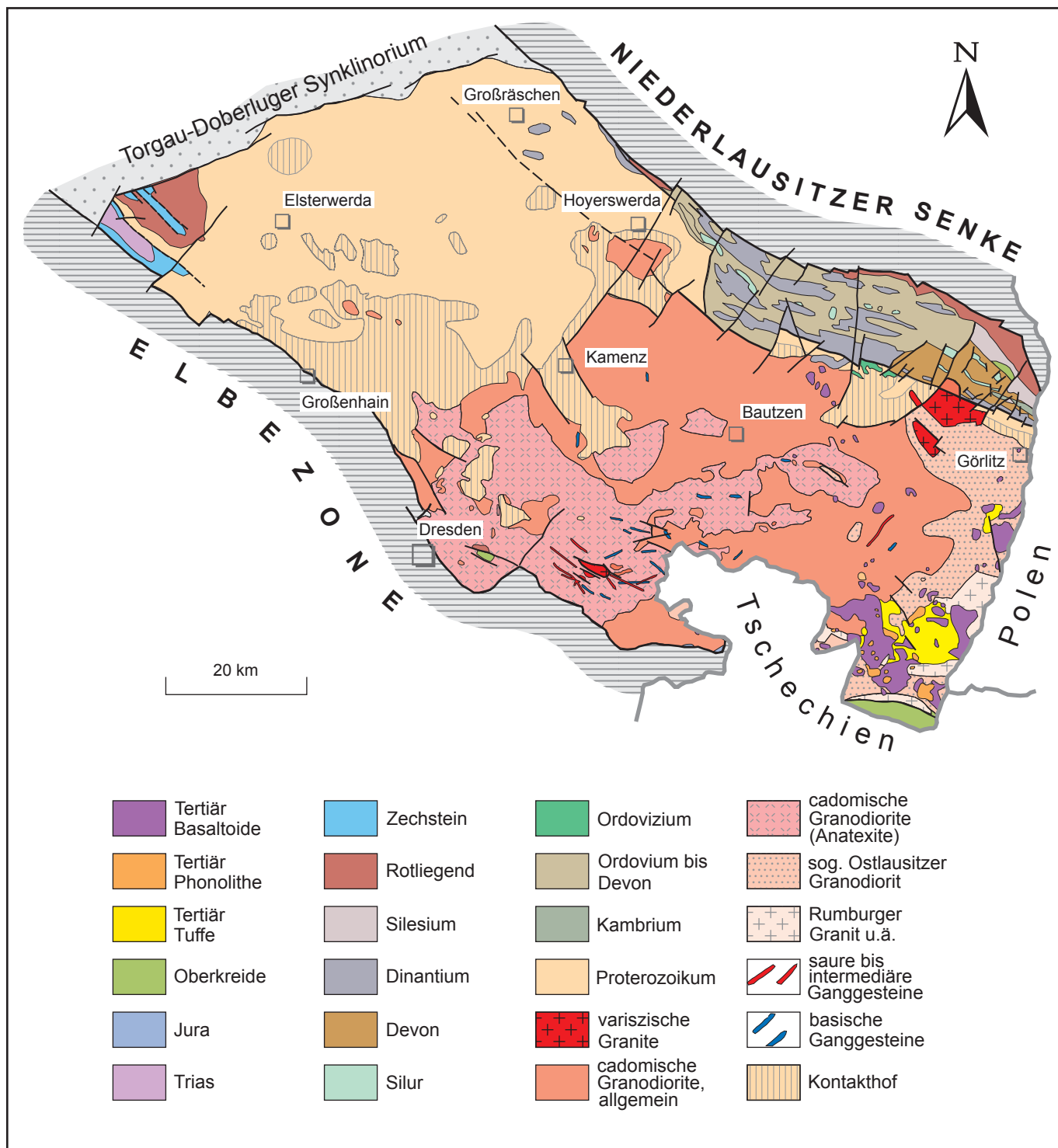
Abb. 40 Geologie des Lausitzer Antiklinoriums Darstellung ohne Sedimente des Känozoikum
