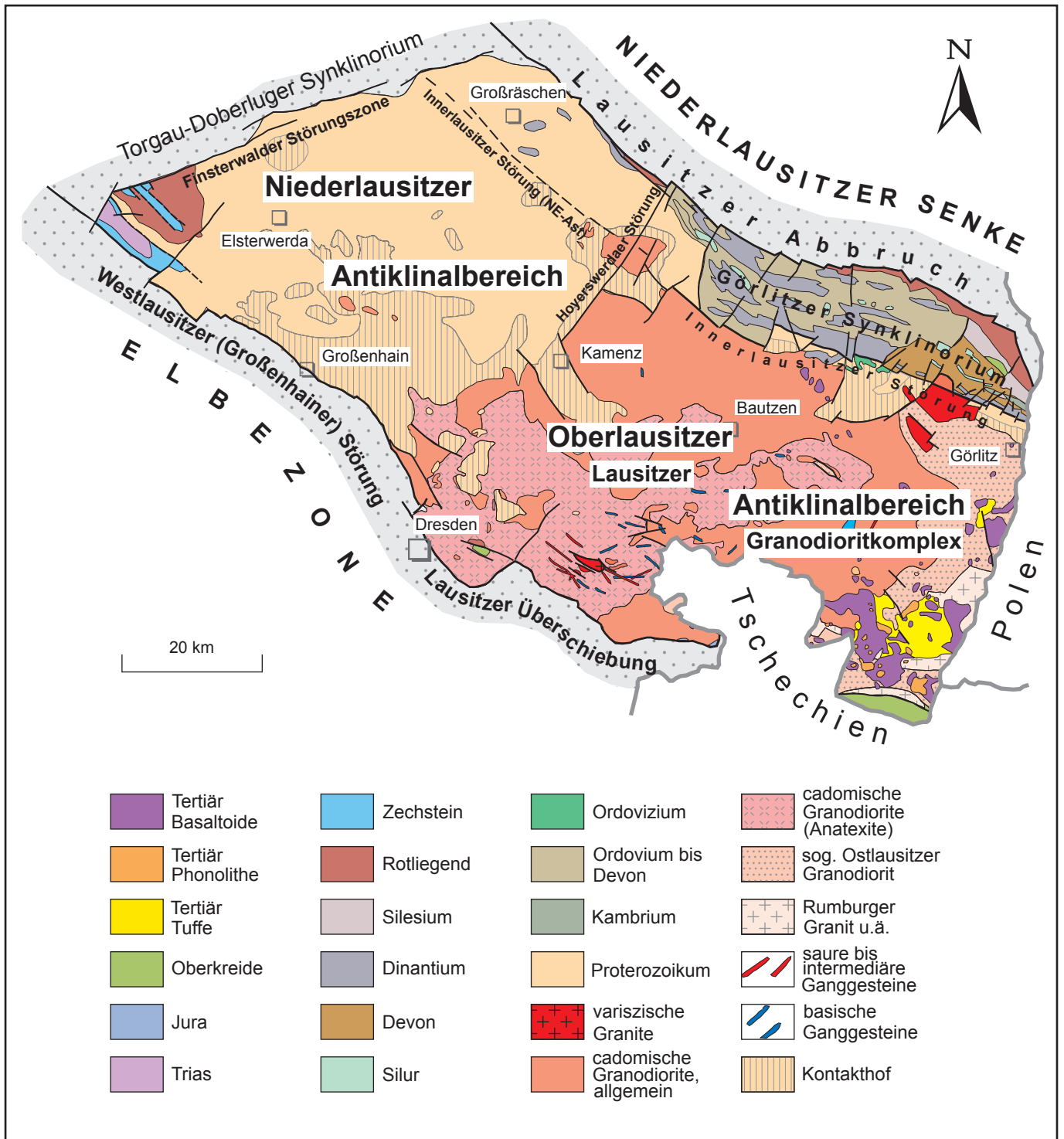
Abb. 40.1 Bedeutende Strukturelemente im Bereich des Lausitzer Antiklinoriums Darstellung ohne Sedimente des Känozoikum
