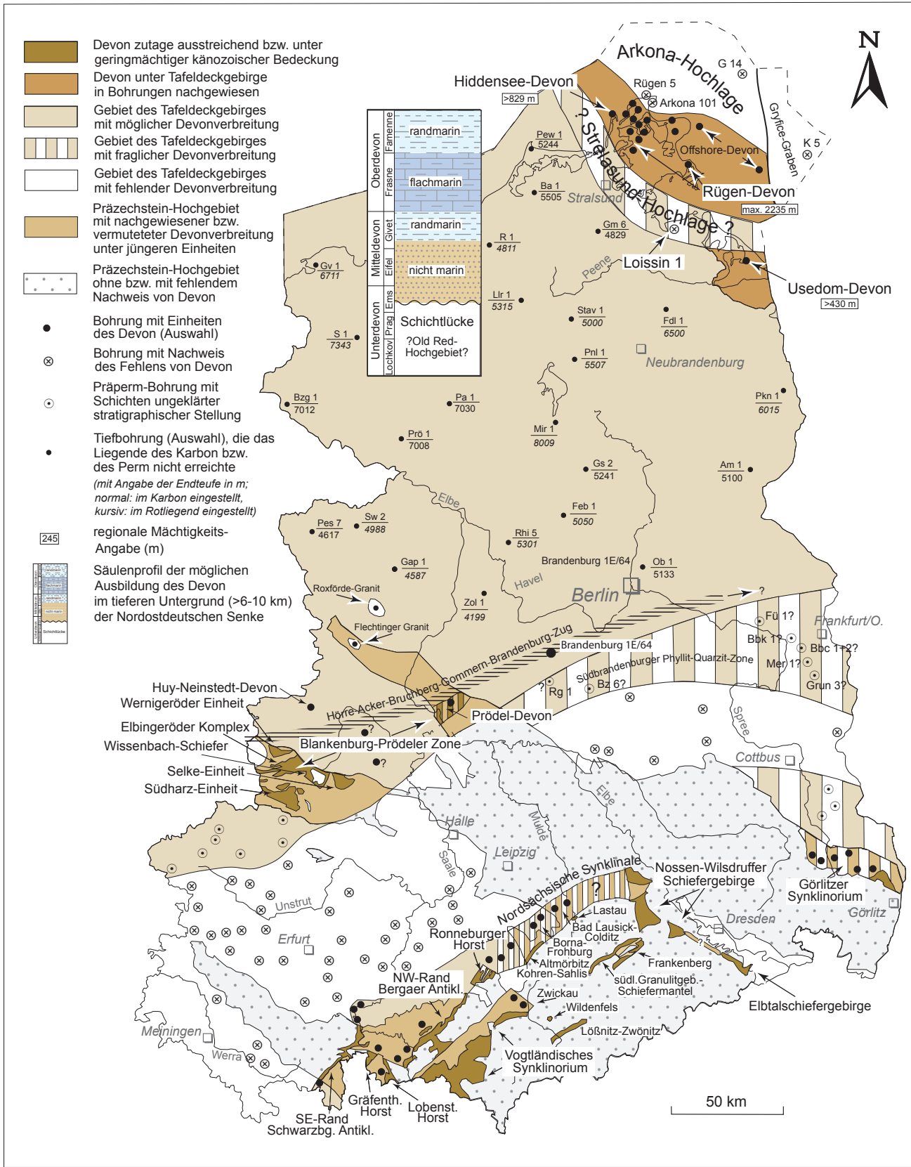
Abb. 6 Heutige Verbreitung von Ablagerungen des Devon in Ostdeutschland
