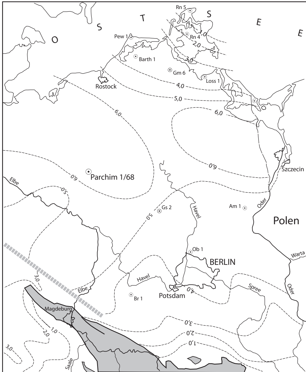
Abb. 1 Lage der Forschungsbohrung Parchim 1/68 (Isolinien dokumentieren die Oberfläche des Präperms)
